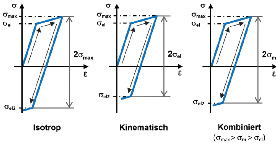
Bild 1 Isotrop, kinematischer und kombinierter Verfestigungsmechanismus
